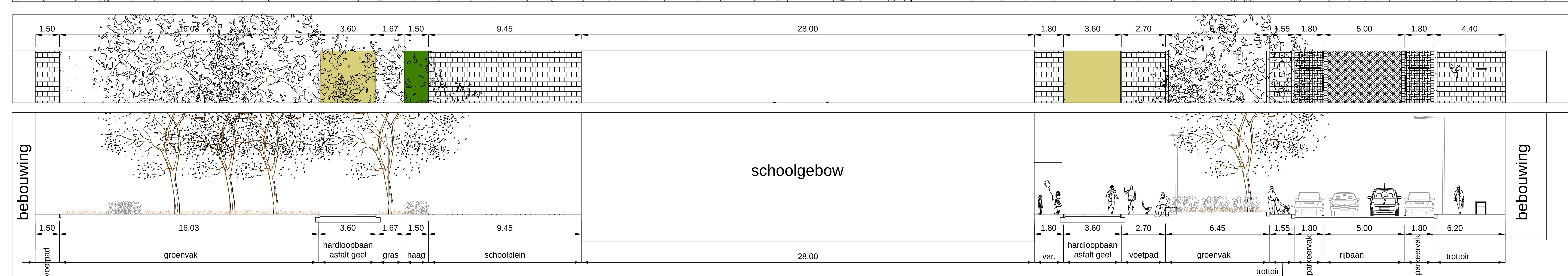
straatbaksteen rood-gederuceerd (kv) straatbaksteen rood-gederuceerd (lv) markering wit boomkran trottoirband 18/20 x 25 cm. "Rotterdam" lage beplanting met accenten betontegels "Rotterdam" 30 x 30 x 4,5 cm. opsluitband 8x20cm. "rotterdam" markering (belijning wit), zoals toegepast in openbare sportplek Roel langerak asfalt geel; Colorfalt design iuxeroxide geel pigment
